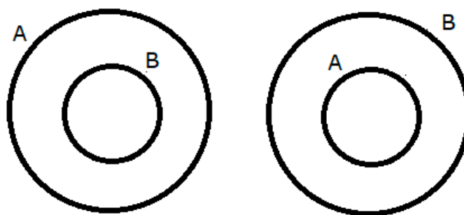
Figura 9: Subconjuntos como um caso particular da intersecção
