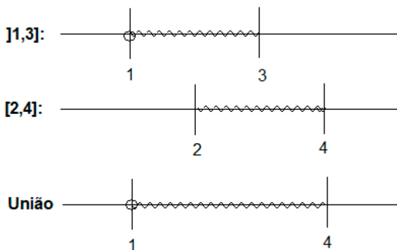
Figura 26: União de Intervalos
