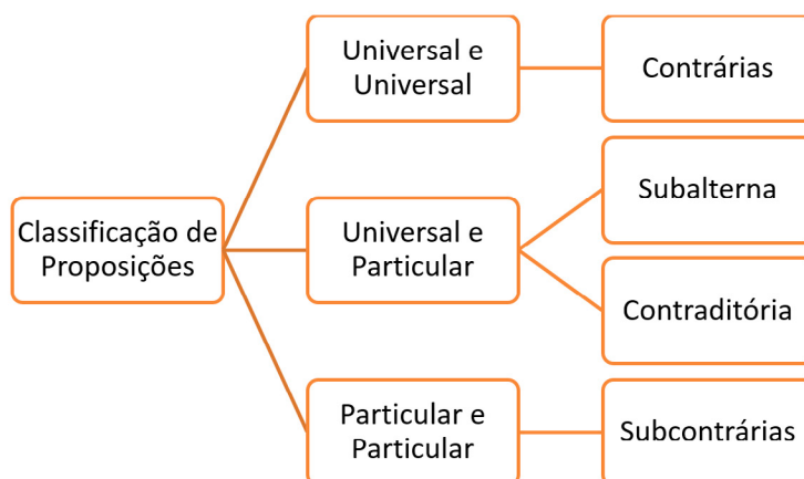
Figura 7: Classificação das Proposições Categóricas
