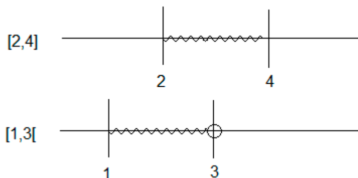
Figura 23: Exemplos de Intervalos
