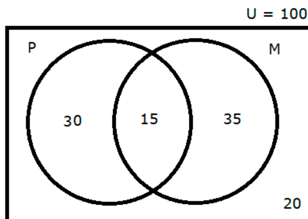
Figura 13: Todo conjunto é subconjunto do Conjunto Universo
