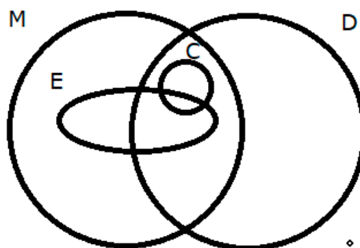
Figura 14: Diagrama de Venn Geral
