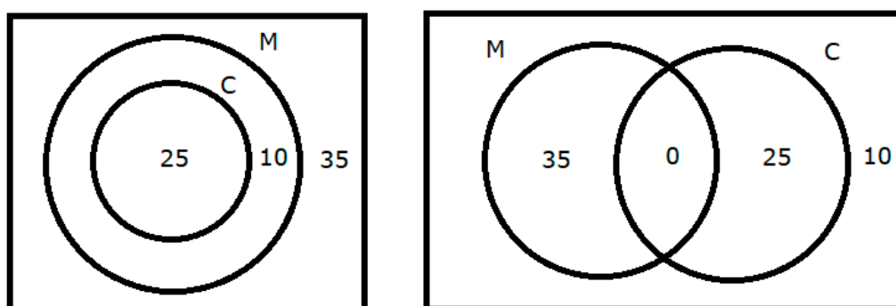
Figura 22: Limites para o Conjunto União e Intersecção quando a Soma do Número de Elementos dos dois conjuntos é menor que o Conjunto Universo
