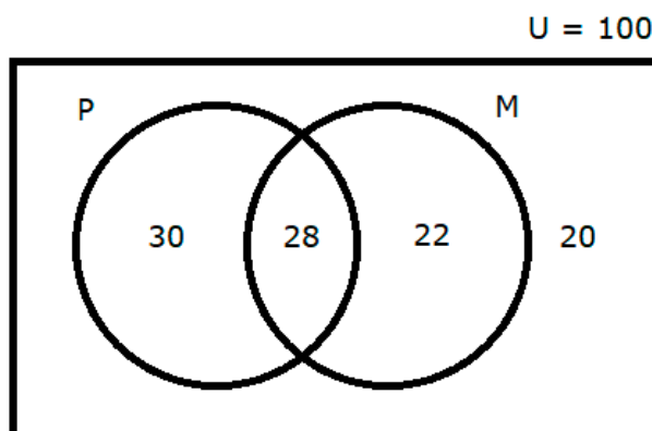
Figura 1: Diagrama de Venn
