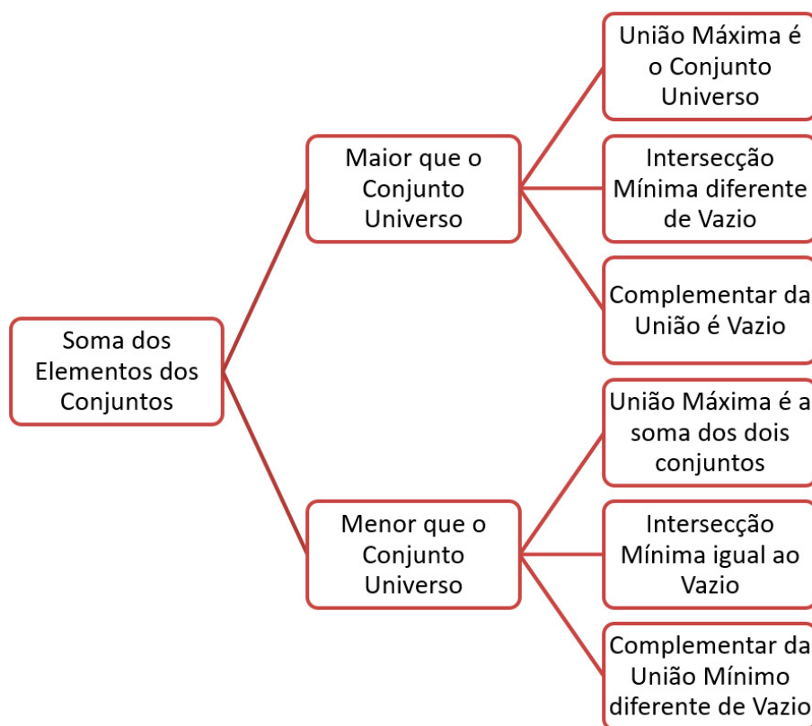
Figura 20: Regras para Reconhecer os Limites da União e Intersecção de Dois Conjuntos
