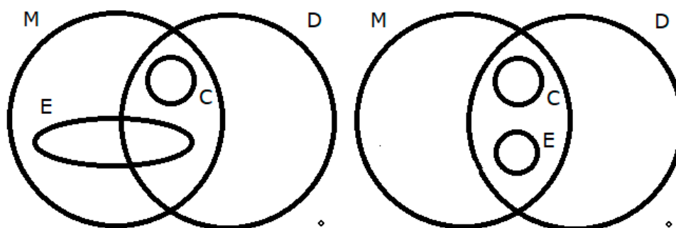
Figura 15: Outras Possibilidades de Diagrama de Venn a serem explorados em questões de prova
