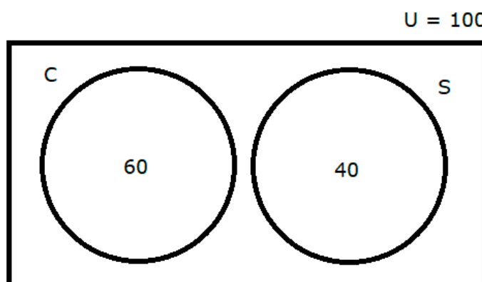
Figura 18: Conjuntos de Pessoas Casadas e Solteiras
