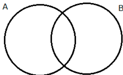
Figura 19: Diagrama da União de Dois Eventos
