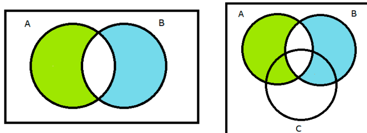
Figura 10: Diferenças entre dois conjuntos no Diagrama de Venn
