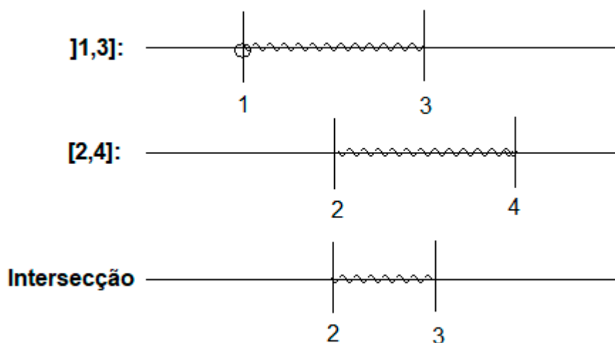
Figura 25: Intersecção em Intervalos
