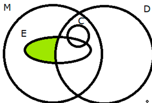
Figura 16: Diagrama de Venn ilustrando uma região em que temos certeza de que existe um elemento
