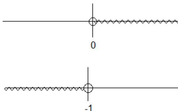
Figura 24: Intervalos incluindo infinidades
