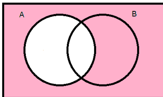
Figura 11: Conjunto Complementar no Diagrama de Venn
