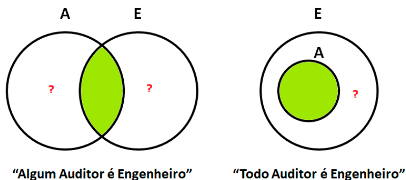
Figura 6: Proposições Subalternas e Superalternas
