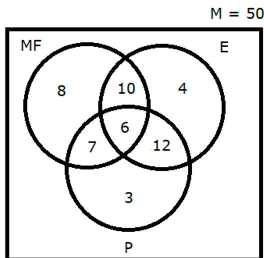
Figura 2: Diagrama de Venn com três conjuntos
