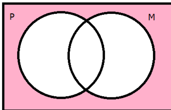
Figura 12: Complementar da União no Diagrama de Venn
