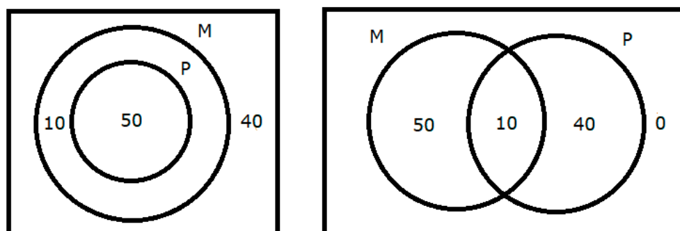
Figura 21: Limites para a União e Intersecção quando a Soma do Número de Elementos dos Dois Conjuntos é maior que o Conjunto Universo
