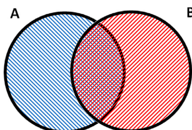
União entre dois Conjuntos
