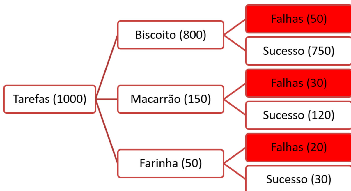
Árvore de Probabilidades
