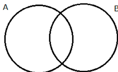
Diagrama da União de Dois Eventos
